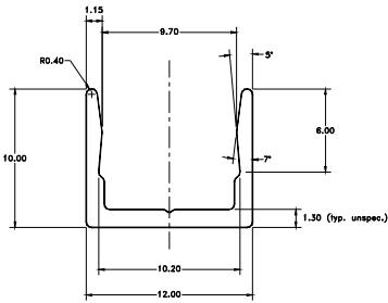
Die: 3753 Channel Min. Order Qty Mtrs:525
